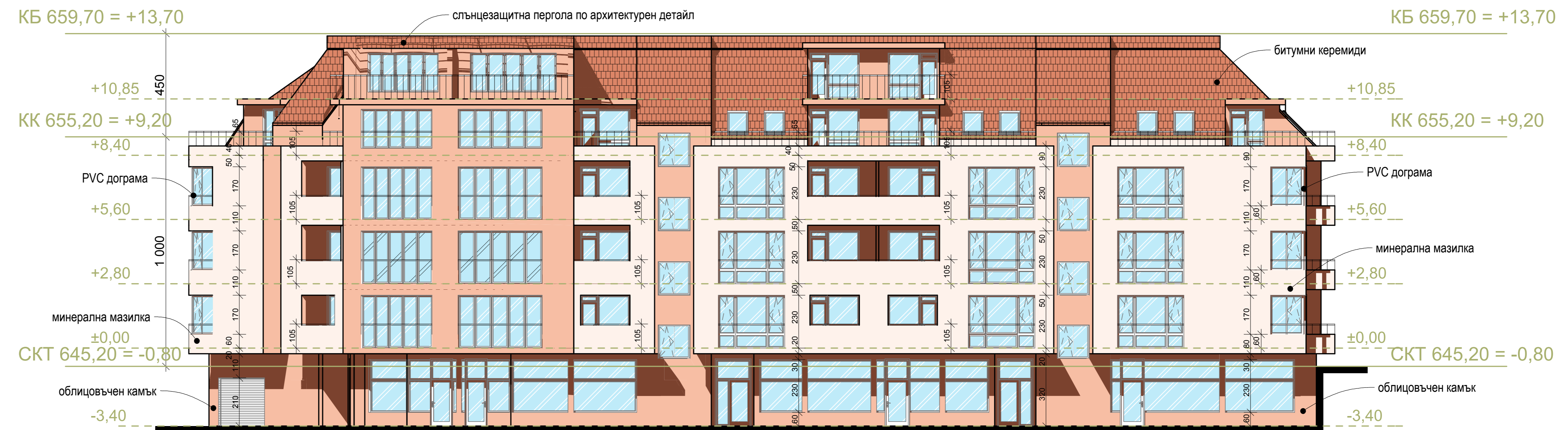
ФАСАДА ЗАПАД, М 1:100
