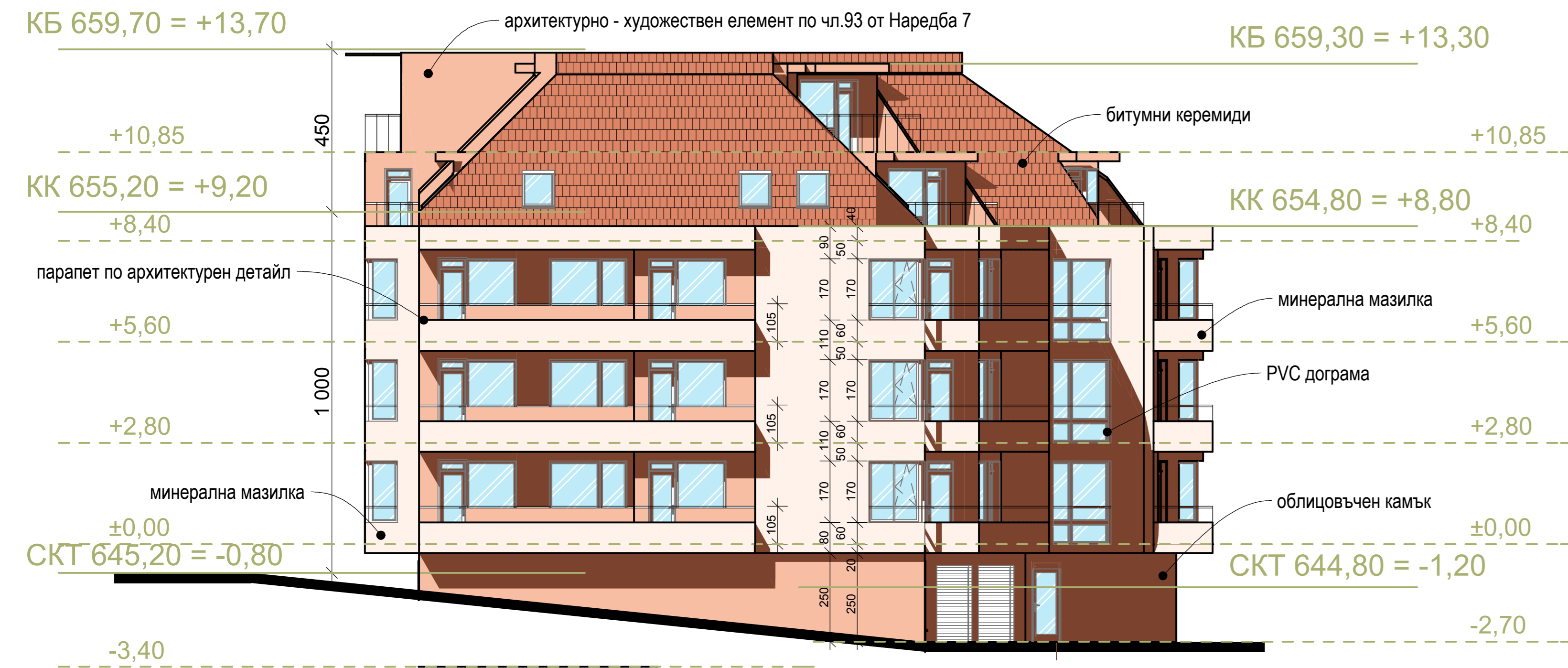
ФАСАДА ЮГ, М 1:100
